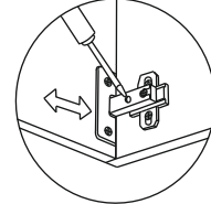
регулировка боковая
